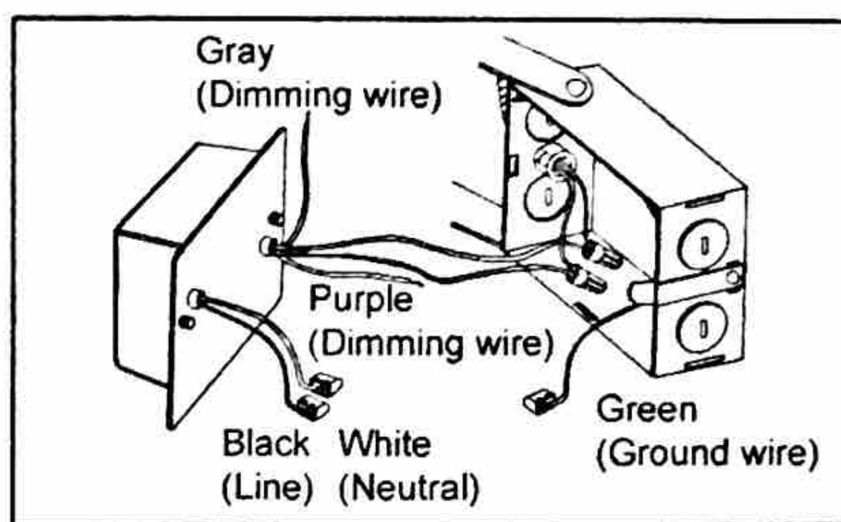
120 / 277V J-Box
