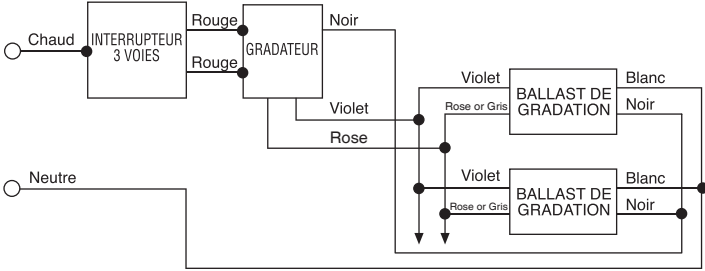
Figure 2 – câblage 3 voies
