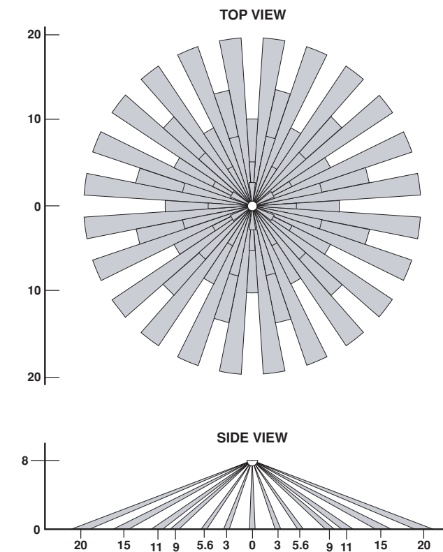
Figura 3 (No. de Cat. OSC15) Rangos del Campo de Visión
