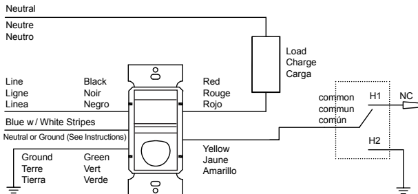
Figure 5: 3-Way Configuration / Figure 5 : Configuration à 3 voies
