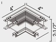
FG-RTL-ACC-3
